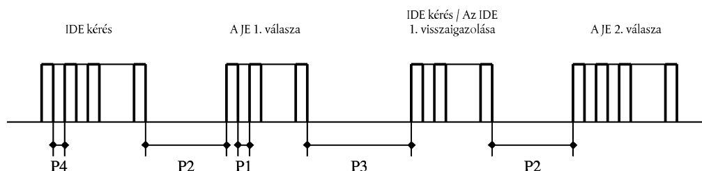
Üzenetáramlás, szinkronizálás
